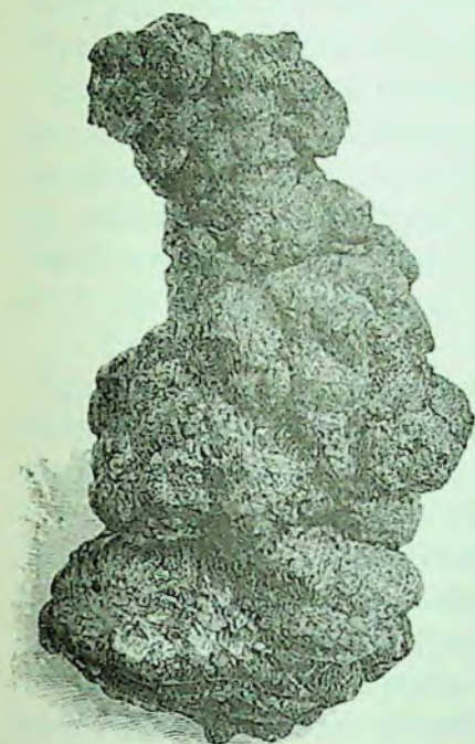
Thurmformiger Erdhaufen von Geophagus Darwinii nov. spec. (Stark verkleinert.) Natürliche Größe: 12 Centimeter hoch, 6\frac{1}{2} Centimeter breit. Gewicht 178 Gramm.
